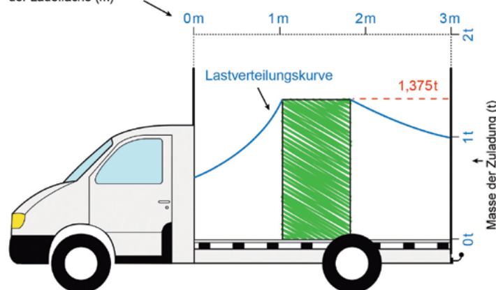
Lastenverteilungsplan für einen Kleintransporter mit einer zulässigen Gesamtmasse bis 3,5 t. Grafik: SVLFG
